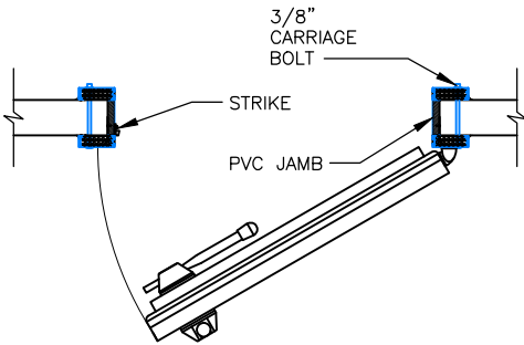
⑮ SCALE: 1/2" = 1'-0"
